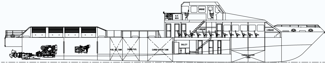
LONGITUDINAL SECTION
